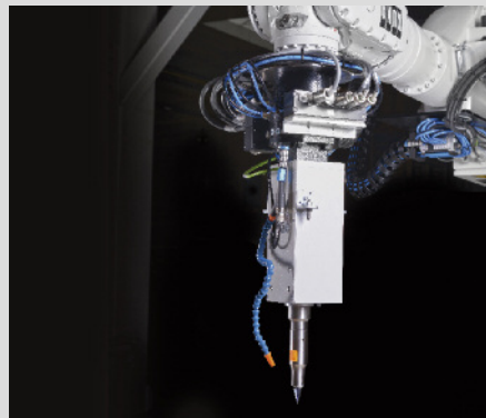
RC 590 Ultraschall schneiden Ultrasound cutting Corte por ultrasonidos
