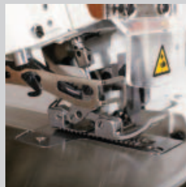
Pied tracteur (5716-86) Pie articulado (5716-86)
