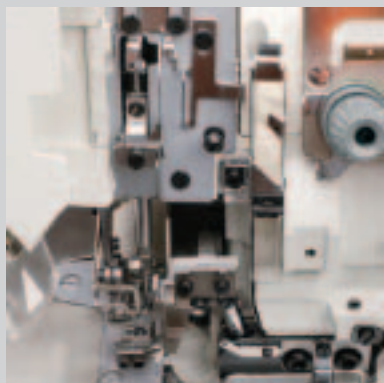
Lubrification de l'aiguille et du fil Lubricación de hilo y aguja
