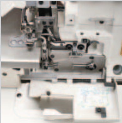
Enfilage simple car les passages des fils sont colorés
